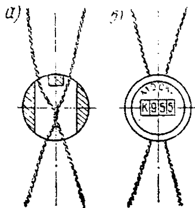
Рис. 2. Схема способа навешивания свинцовых пломб с камерой
