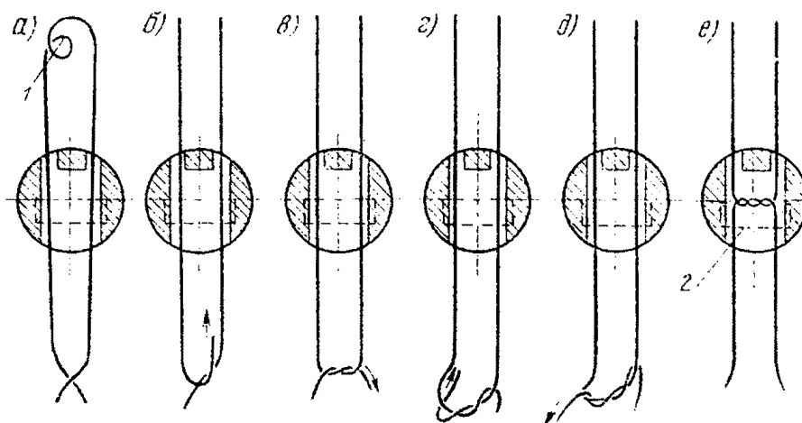
Рис. 3. Схема способа навешивания полиэтиленовых пломб с камерой: 1 — двойная петля вокруг ушков дверной накладки и стойки; 2 — скоба
